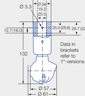
Slip-on connection ASME - BPE 1997 (OD-Tube)
