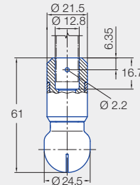
Slip-on connection ASME - BPE 1997 (OD-Tube)
